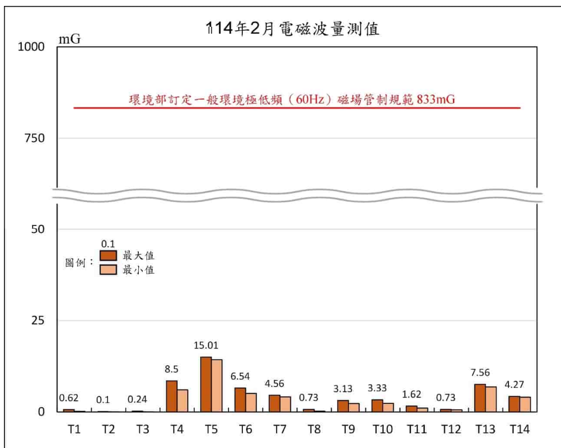
圖 3.1-6 歷次電磁波監測成果
