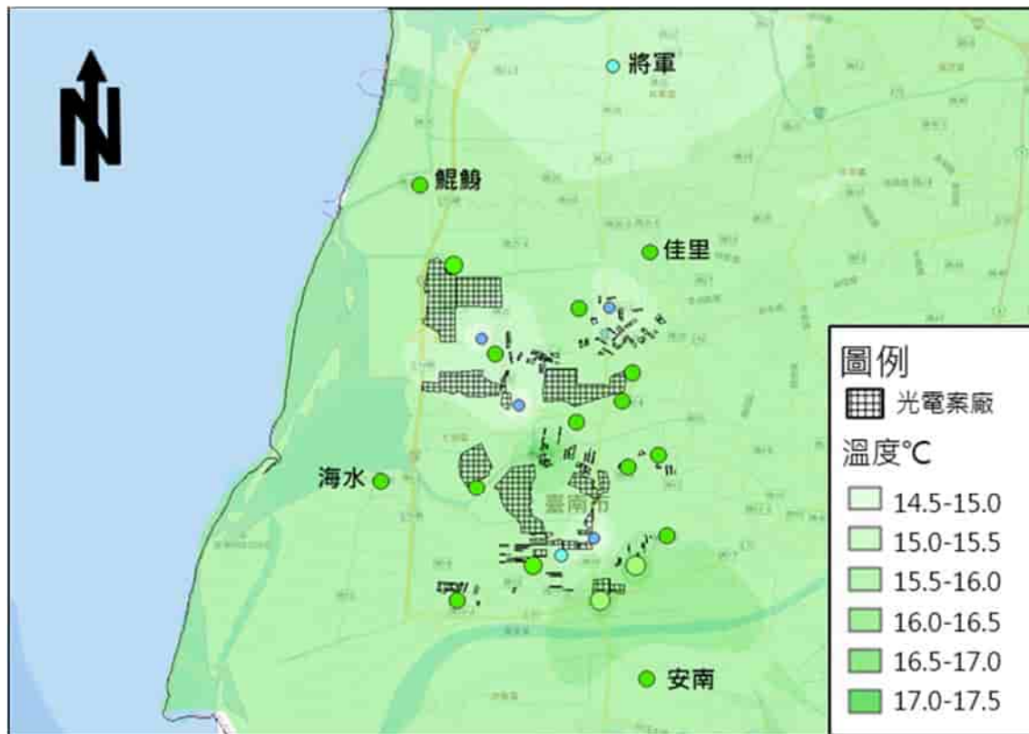
圖 3.1-1 一月平均溫度分布示意圖
