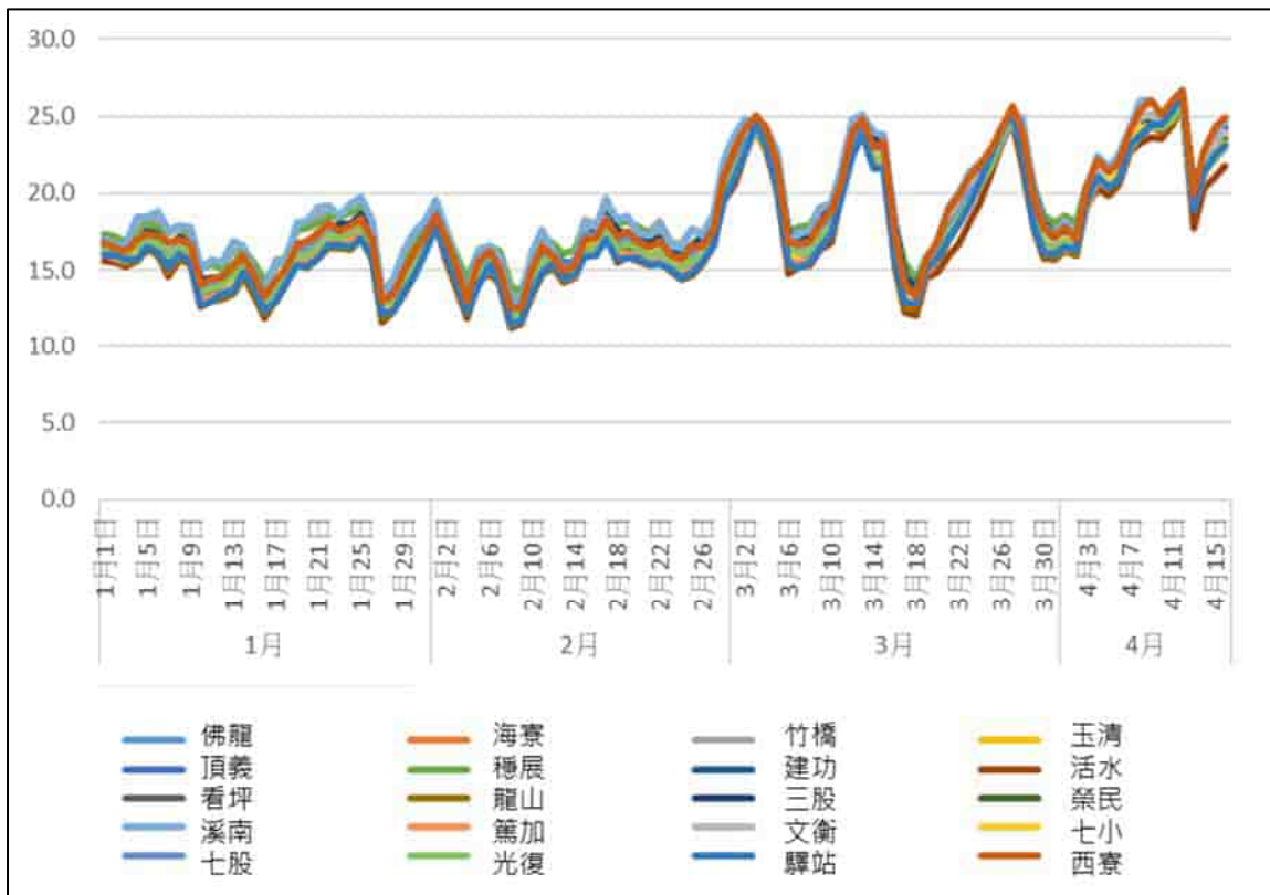
圖 2.2-2 本季各測站溫度監測成果
