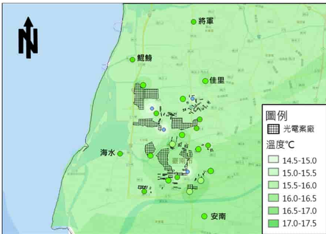
圖 3.1-3 三月平均溫度分布示意圖
