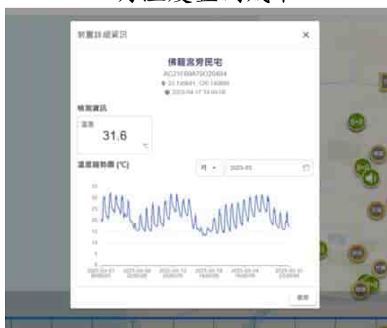
三月溫度監測成果
