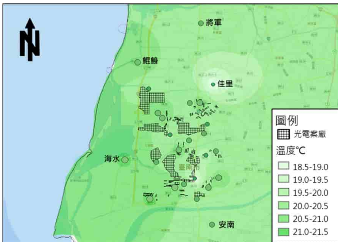
圖 3.1-4 四月平均溫度分布示意圖
