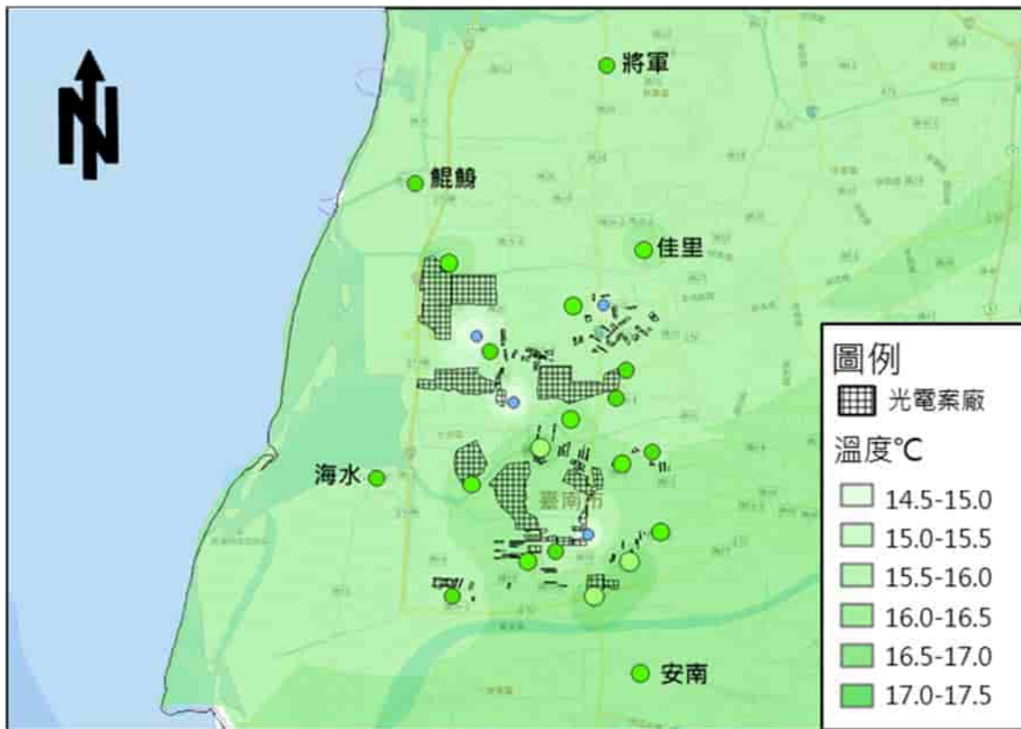
圖 3.1-2 二月平均溫度分布示意圖
