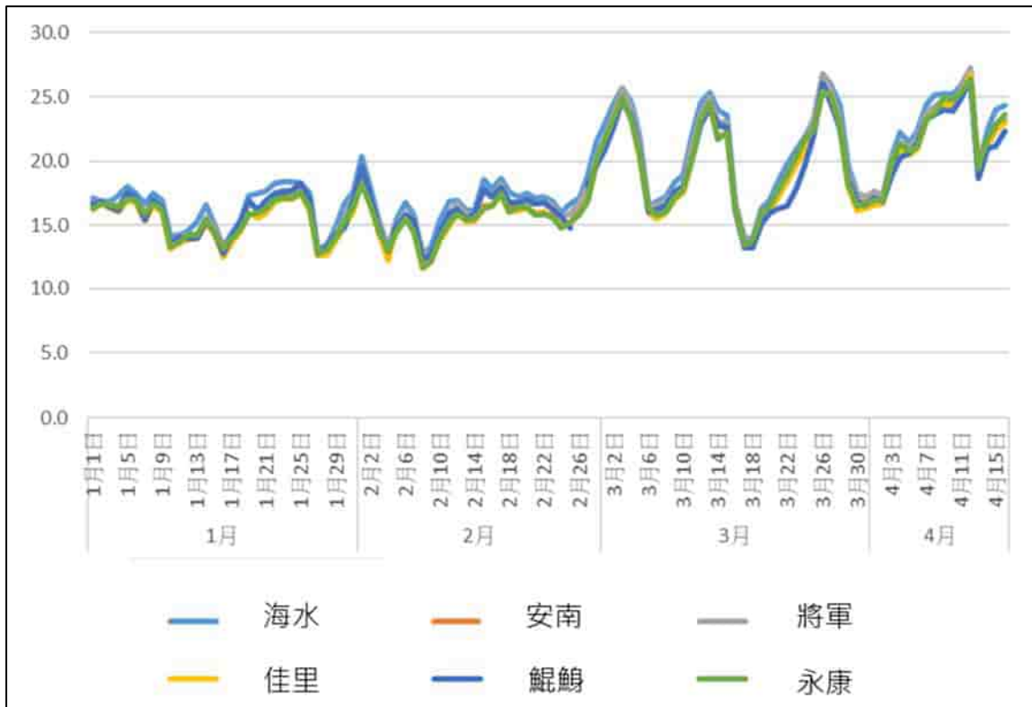
圖 2.2-1 本季中央氣象署溫度監測成果
