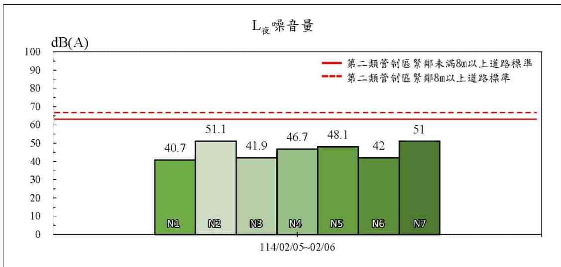
圖 3.1-5 歷次環境噪音監測成果
